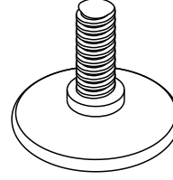
M6 Bingo ayak 4 adet
